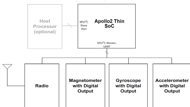
Apollo2 Thin SoC 典型传感应用电路图
