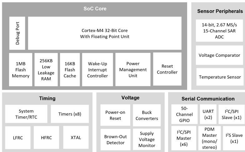
Apollo2 Thin 超低功耗 SoC 结构框图
