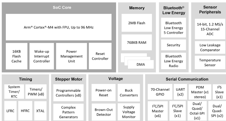
超低消費電力Apollo3 Blue Plus SoCのブロック図
