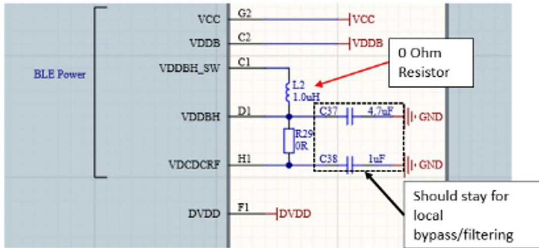
Figure 14-1: BLE Inductor
